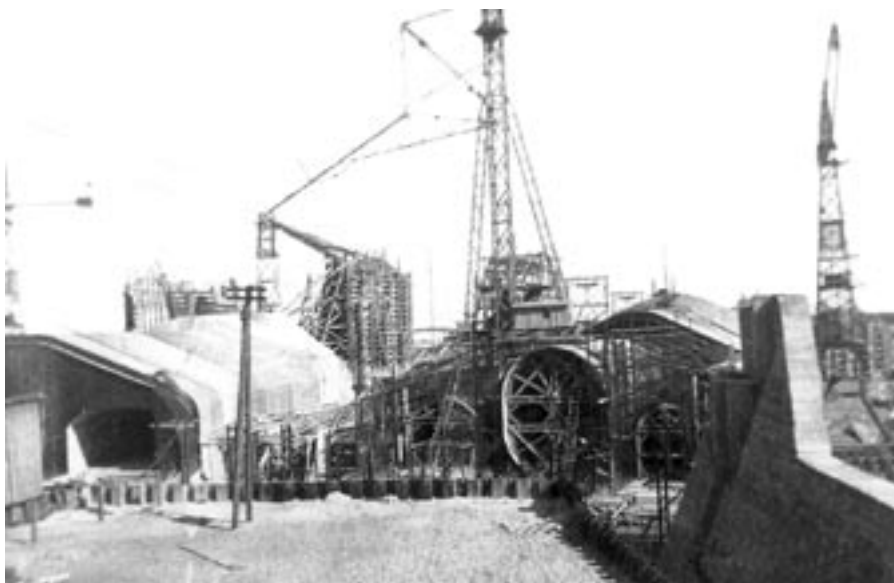
1. Budowa śluzy i elektrowni na zaporze czołowej.
